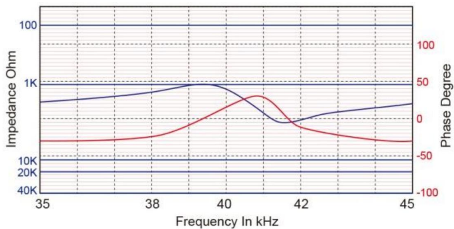
图 2：阻抗幅度/相位
