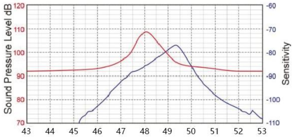
图 3: 声压灵敏度
