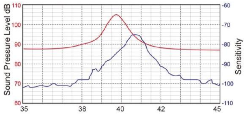
图 3: 声压灵敏度
